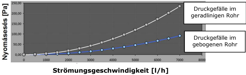
Diagramm 2 – Druckgefälle im rostfreien Wärmetauscher
